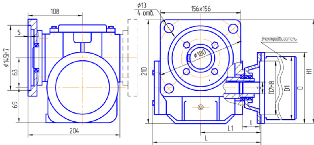
Вариант сборки 56(возможны все варианты сборок), вариант крепления 3(4), вариант расположения червячной пары 1
