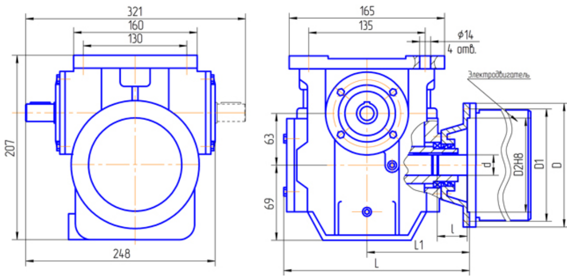
Вариант сборки 52(51,53,56,61,62,63,66), вариант крепления 2, вариант расположения червячной пары 1
