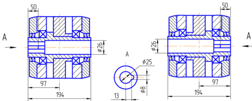
Вариант сборки 56
